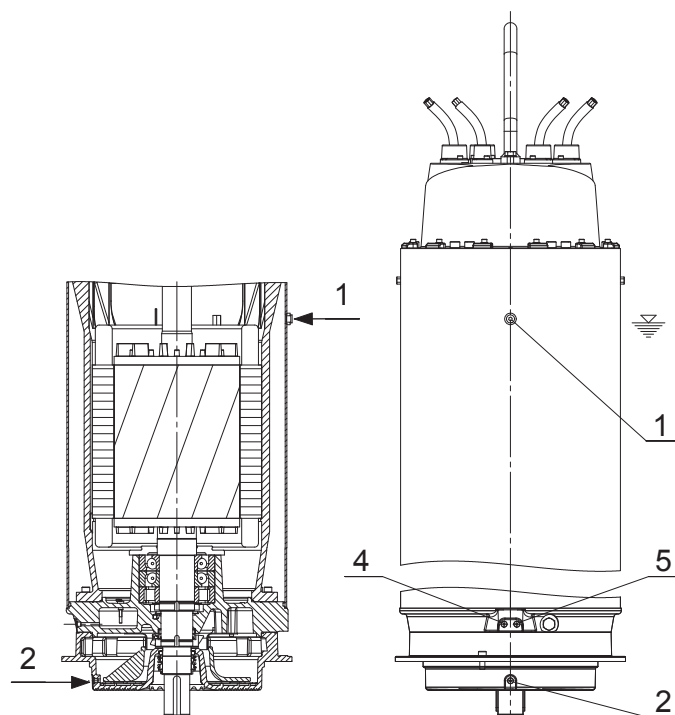
Imaginea 25 Completați și scurgere a lichidului de răcire / lubrifianț XFP PE6 cu manta de răcire
