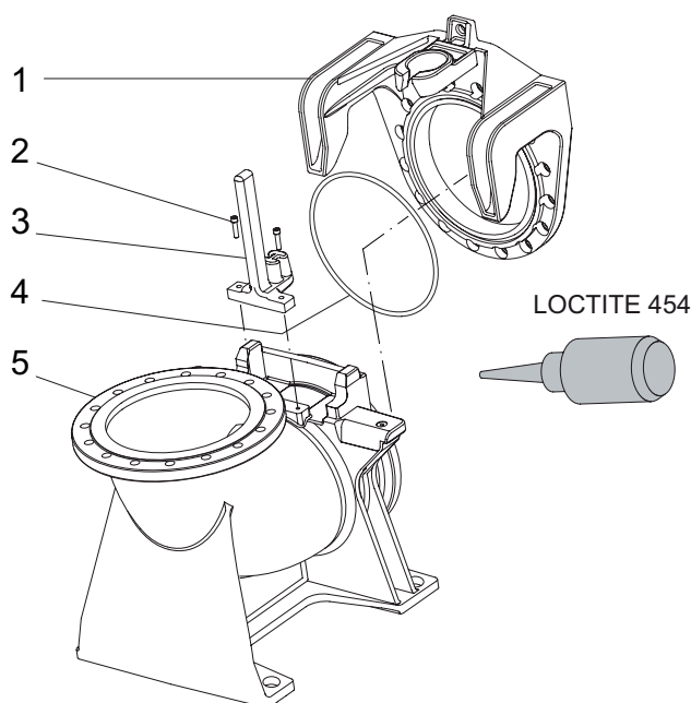
Imaginea 11 Piesa de picior de ÎP DN 100 - 800
