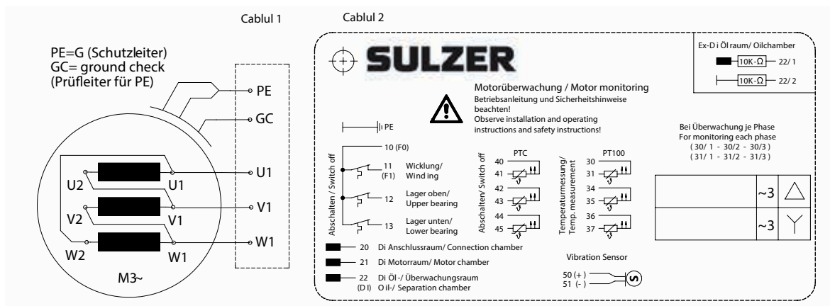
Imaginea 19 Varianta executivă de 60 Hz : Un cablu de racord pentru motor și un cablu de comandă - pentru supravegherea optimă a motorului
