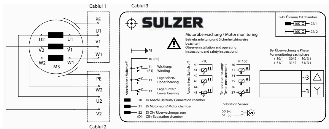
Imaginea 18 Variante specială: două cabluri de racord ale motorului și un cablu de comandă - pentru supravegherea optimă a motorului
