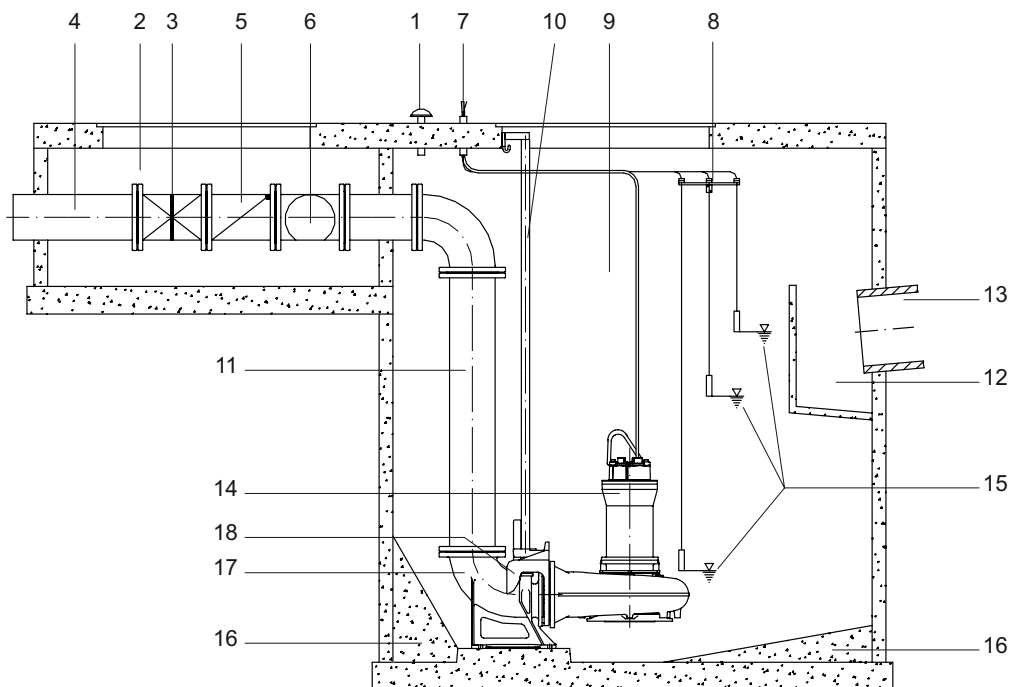
Imaginea 10 Instalare umedă, verticală cu sistem automat de cuplare Sulzer
