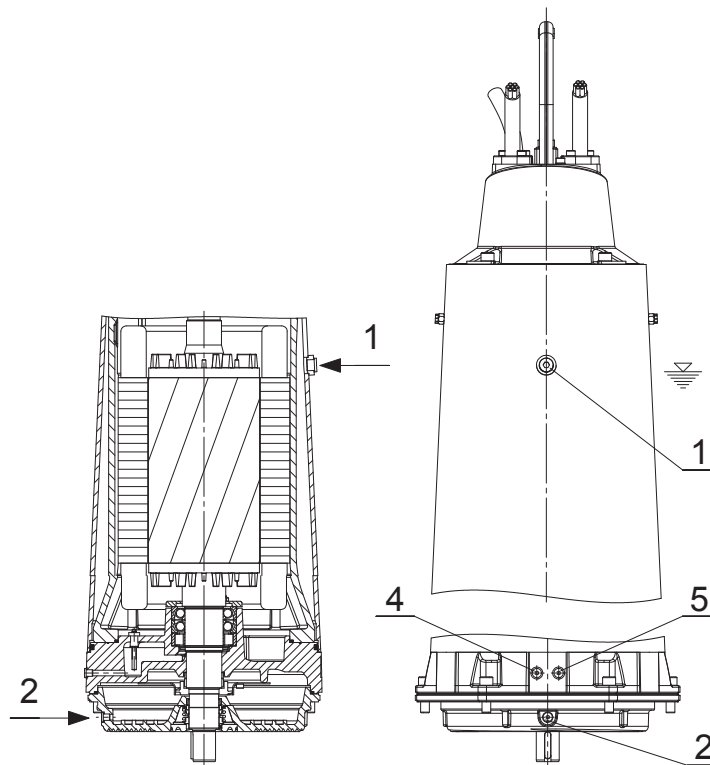
Imaginea 24 Completați și scurgere a lichidului de răcire / lubrifiant XFP PE4 - PE5 cu manta de răcire
