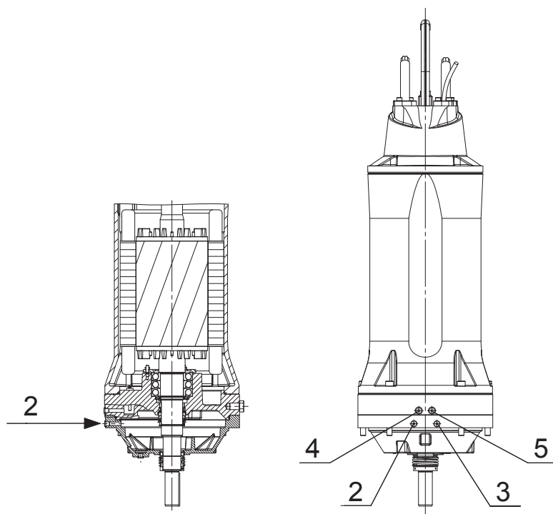
Imaginea 26 Completați și scurgere a lichidului de răcire / lubrifianț VUPX / AFLX PE4 - PE5
