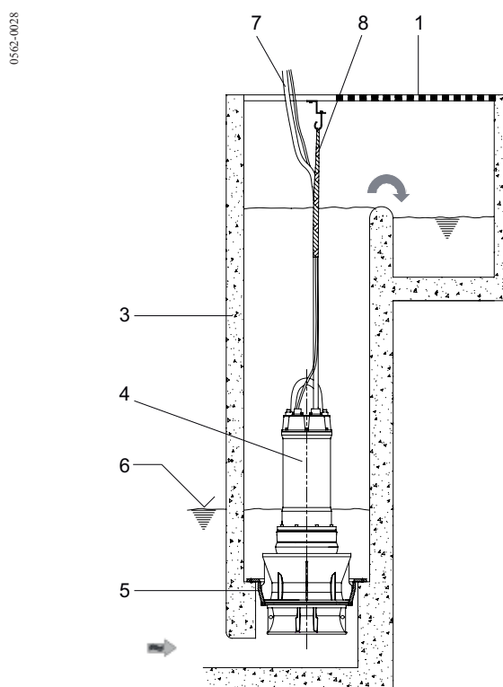
Imaginea 13b AFLX/VUPX într-un cămin din beton
