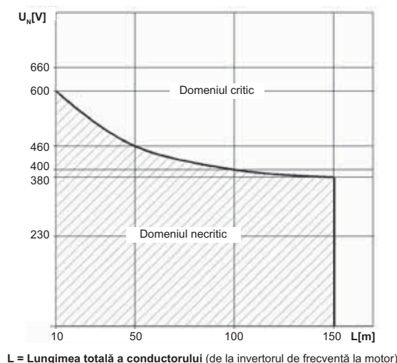
Imaginea 9 Domeniul critic/necritic
