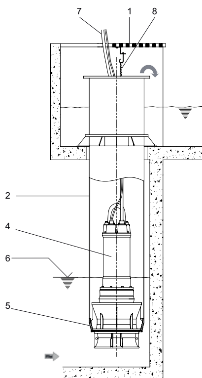
Imaginea 13a AFLX/VUPX în tub de presiune din oțel
