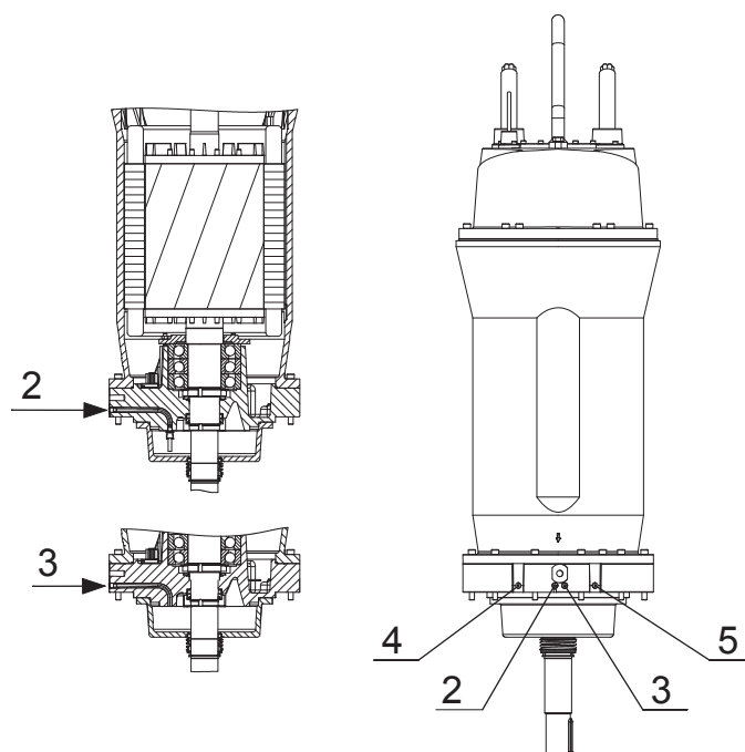
Imaginea 27 Completați și scurgere a lichidului de răcire / lubrifianț VUPX / AFLX PE6
