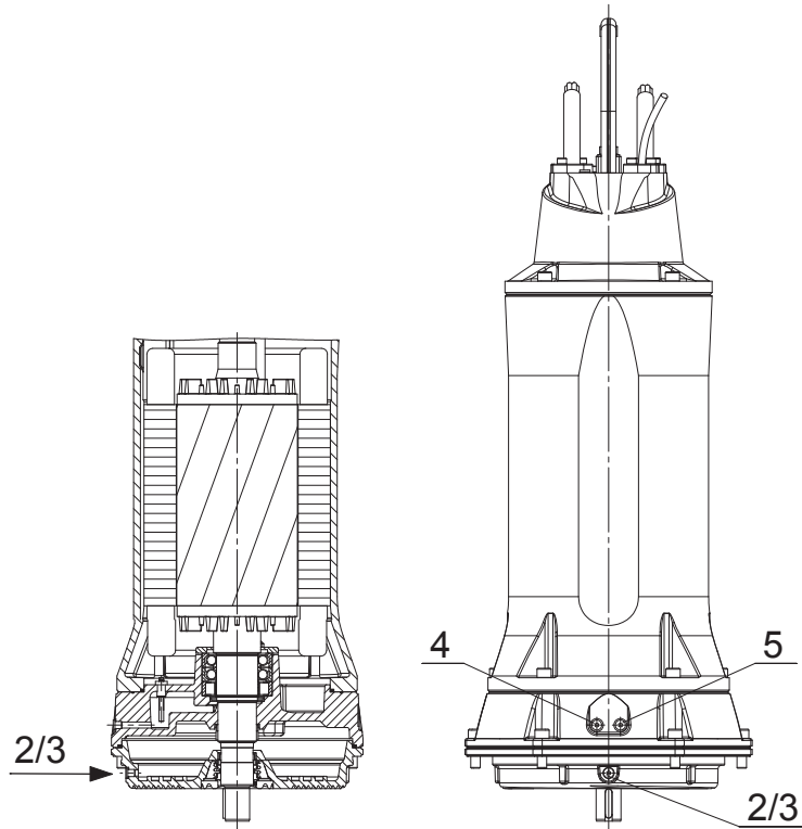
Imaginea 23 Completați și scurgere a lichidului de răcire / lubrifiant XFP PE4 - PE5 fără manta de răcire
